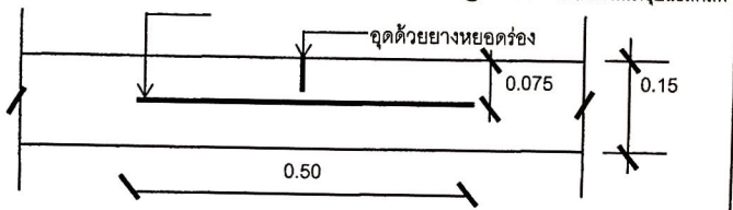
CONTRACTION JOINT (ทุกระยะ 5.00 เมตร)
