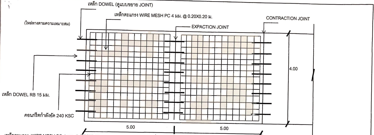
แปลนการวางตะแกรงเหล็ก
